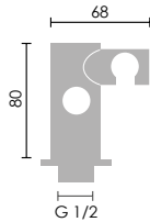
123213OR Codo de ducha 1/2 con soporte, redondo PVP: 36,00 €
