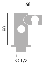
123213NG Codo de ducha 1/2 con soporte, redondo PVP: 36,00 €
