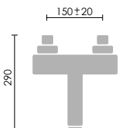
121308 Monomando fregadero pared caño fundido (13x17) / Wall sink mixer
