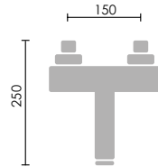
121314 Monomando fregadero pared caño alto (13x17) / Wall sink mixer
