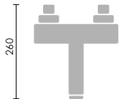
121407 Batería fregadero pared (13x17) / Wall sink mixer Acabado cromo Montura cerámica 1/4 v Aireador H22 mm. PVP: 95,00 €
