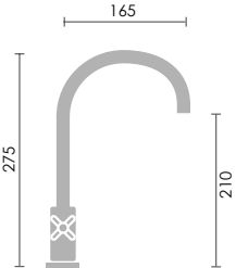
121415 Monobloc fregadero / Mono sink mixer
