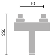
121315 Monomando fregadero pared caño conformado (9x13) / Wall sink mixer
