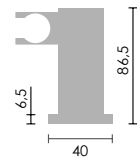
123214NG Codo de ducha 1/2 con soporte, cuadrado PVP: 40,00 €
