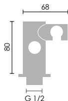
123213RC Codo de ducha 1/2 con soporte, redondo PVP: 36,00 €
